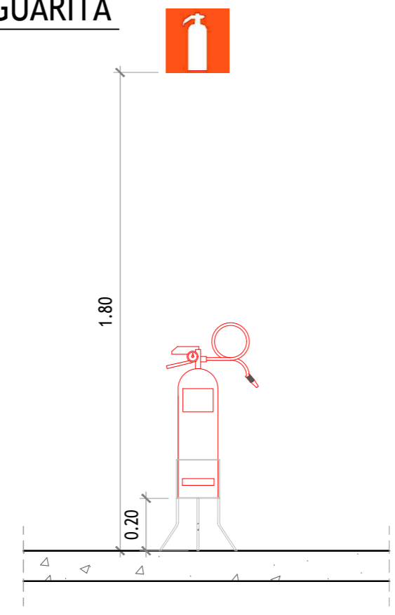
2 CORTE DO EXTINTOR ESCALA 1:20
