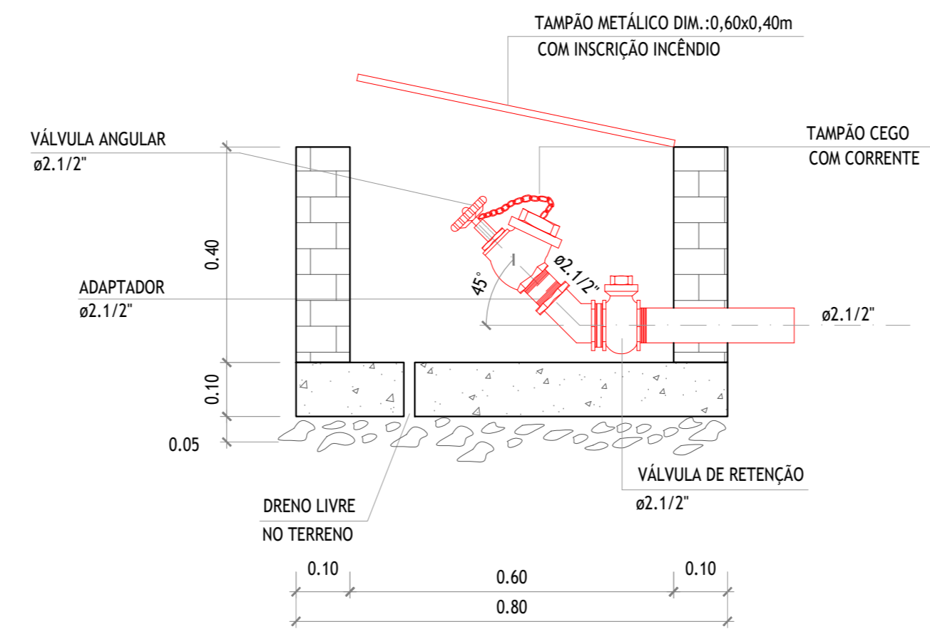
3 HIDRANTE DE PASSEIO ESCALA 1:10
